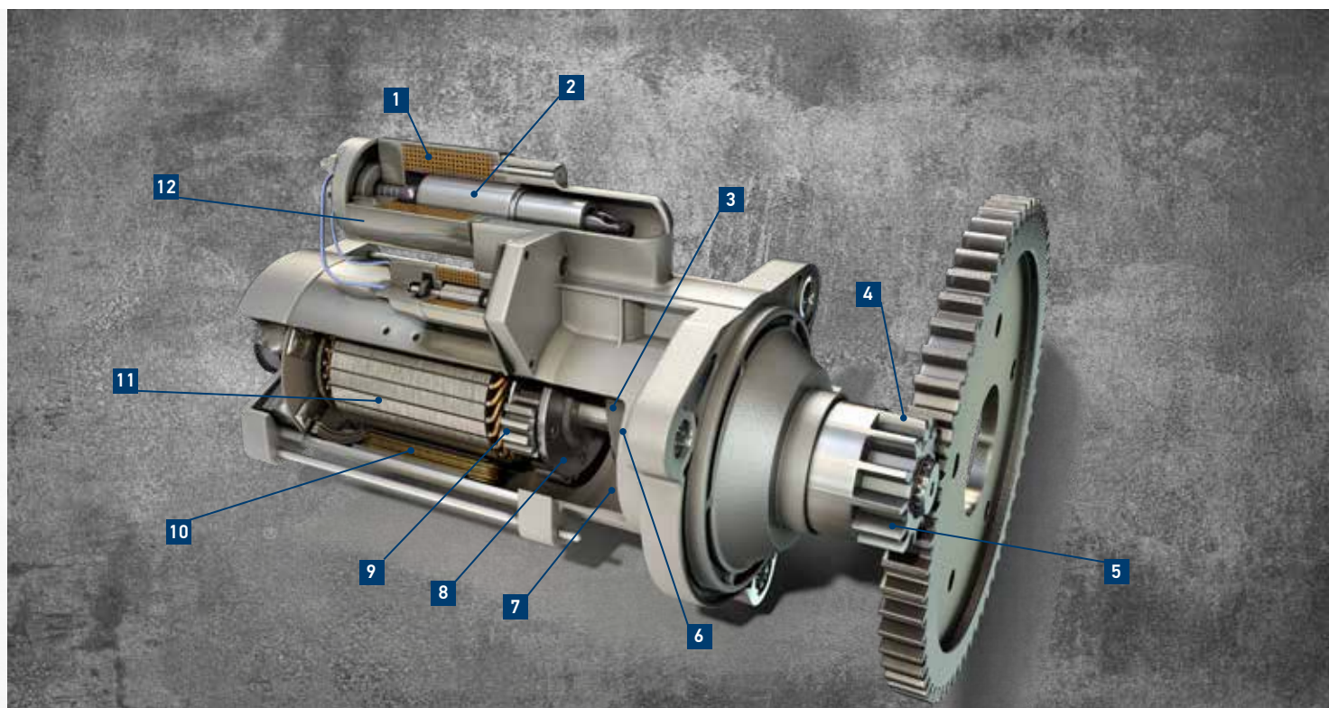
1. Devanado | 2. Tirante | 3. palanca de embrague | 4. Impulsor | 5. Eje de armadura | 6. Leva 7. Engranaje de anillo | 8. Engranaje planetario | 9. Embrague de disco | 10. bobinado | 11. Inducido | 12. Interruptor magnético
